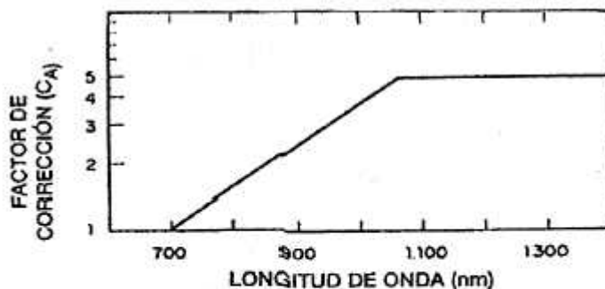
Figura 1. Factor de corrección de los valores TLV para \lambda = 700\text{-}1400 \text{ nm}^*
